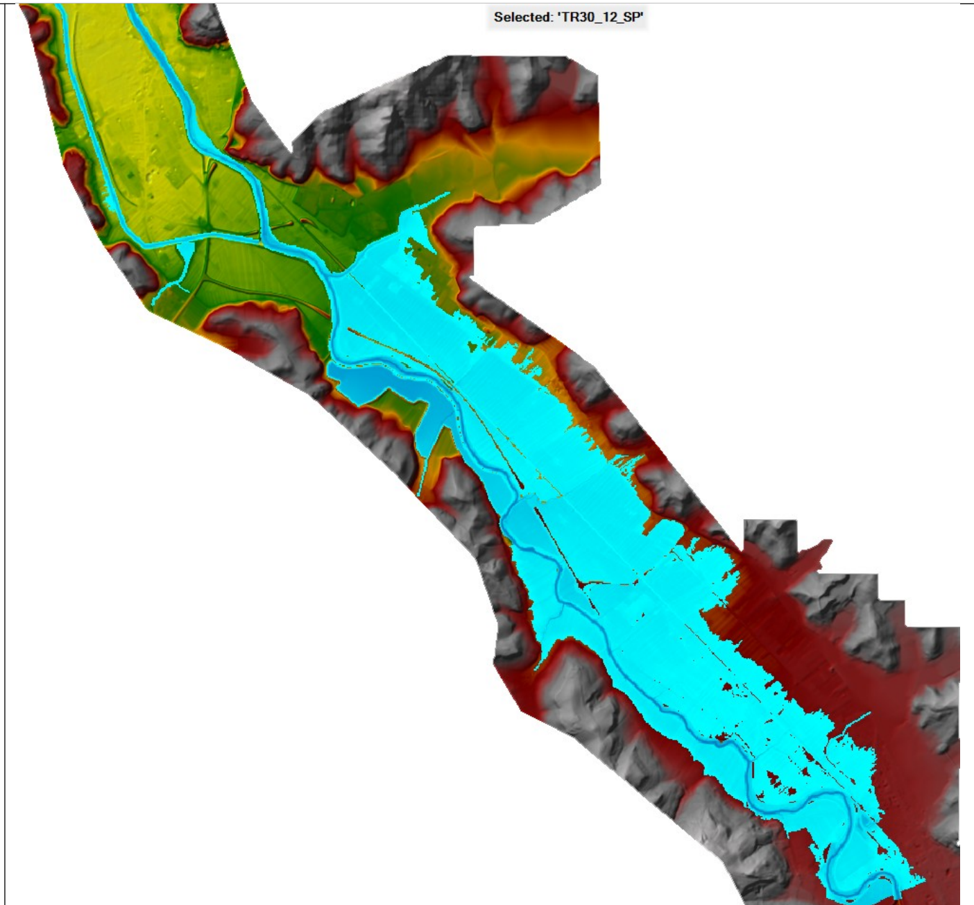
Battenti di inondazione per Tr30 – stato di progetto (12 ore)
