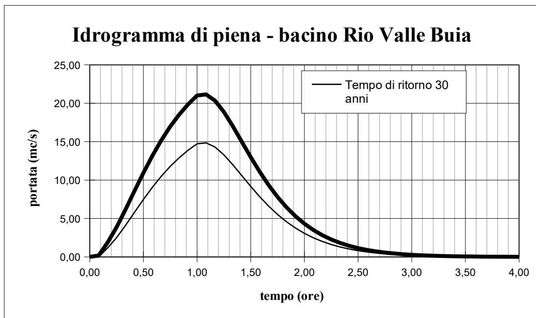
Figura 14 - idrogrammi critici Rio Valle Buia
