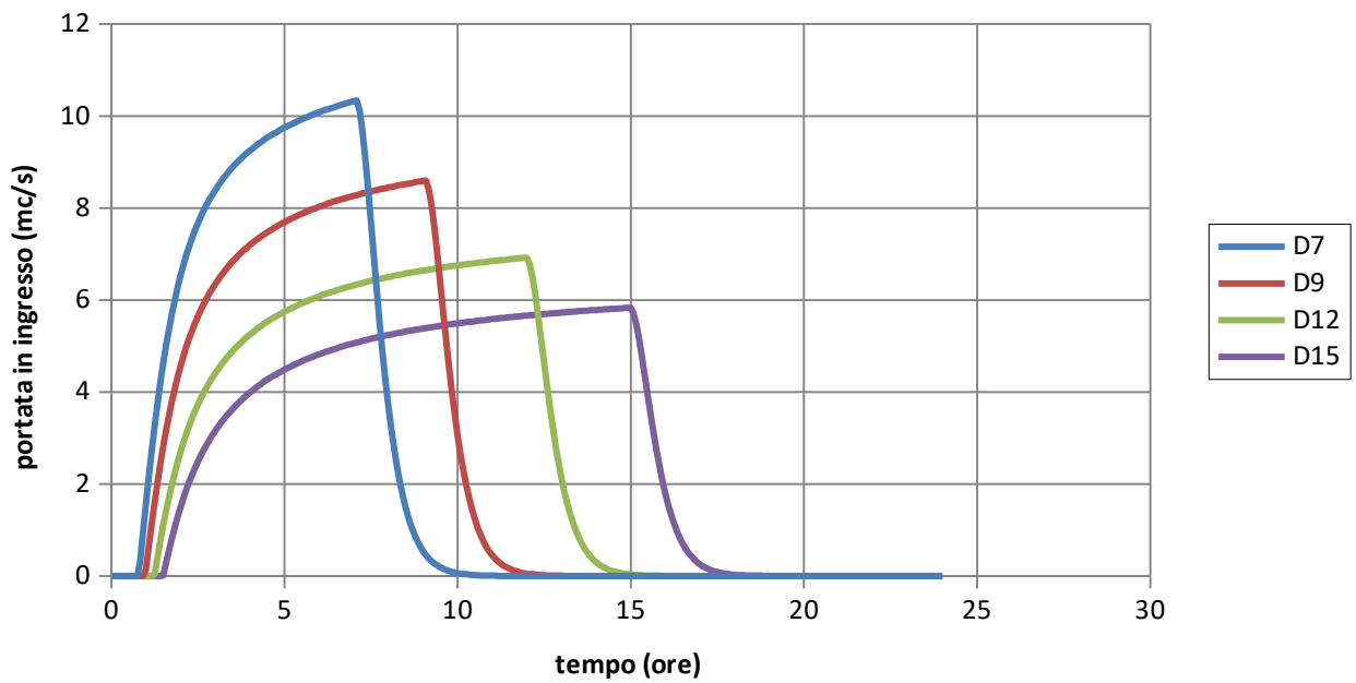
Figura 13 - idrogrammi del Rio Vallone per Tr30
