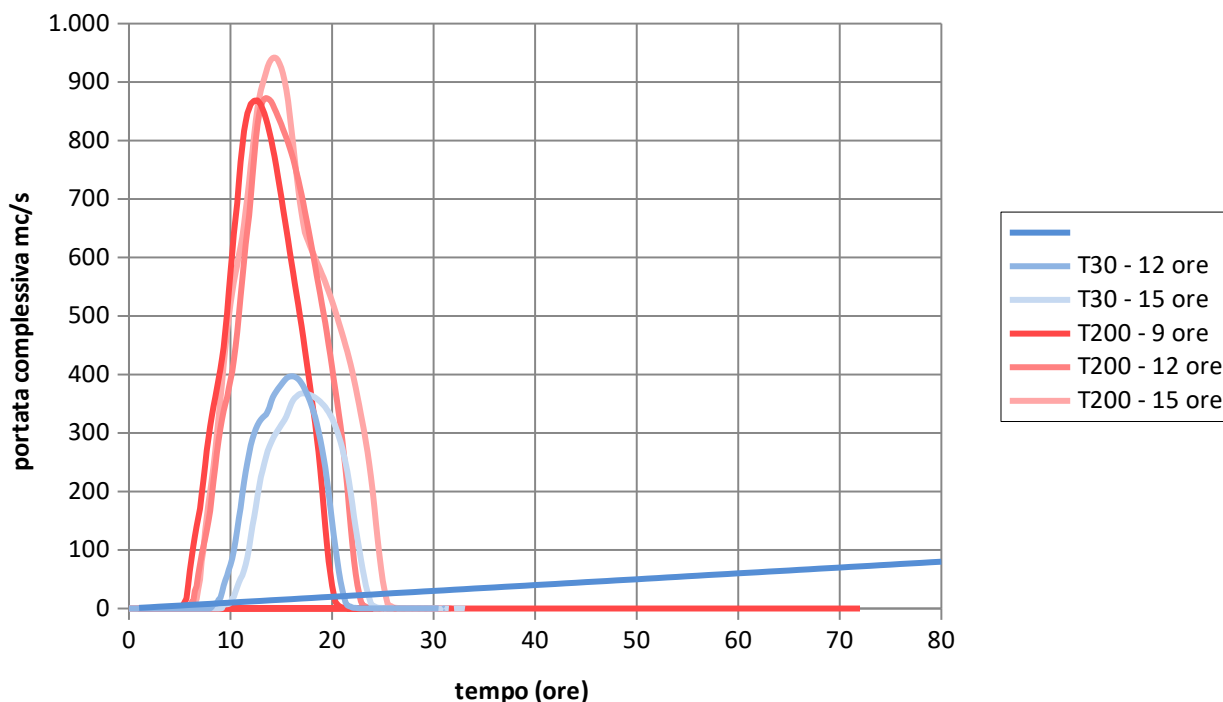
Figura 3 - idrogrammi in ingresso alla sezione di monte - solo parte fuori alveo
