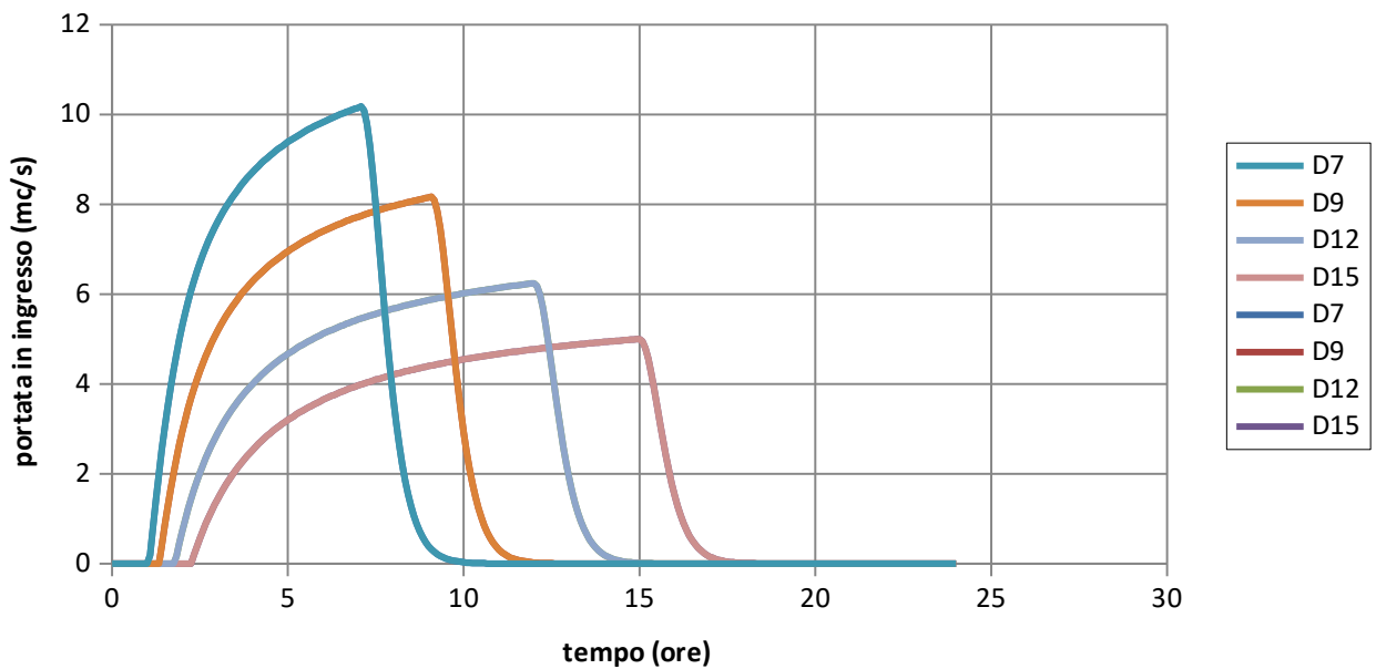
Figura 9 - Idrogrammi del Borro Renaccio per Tr30
