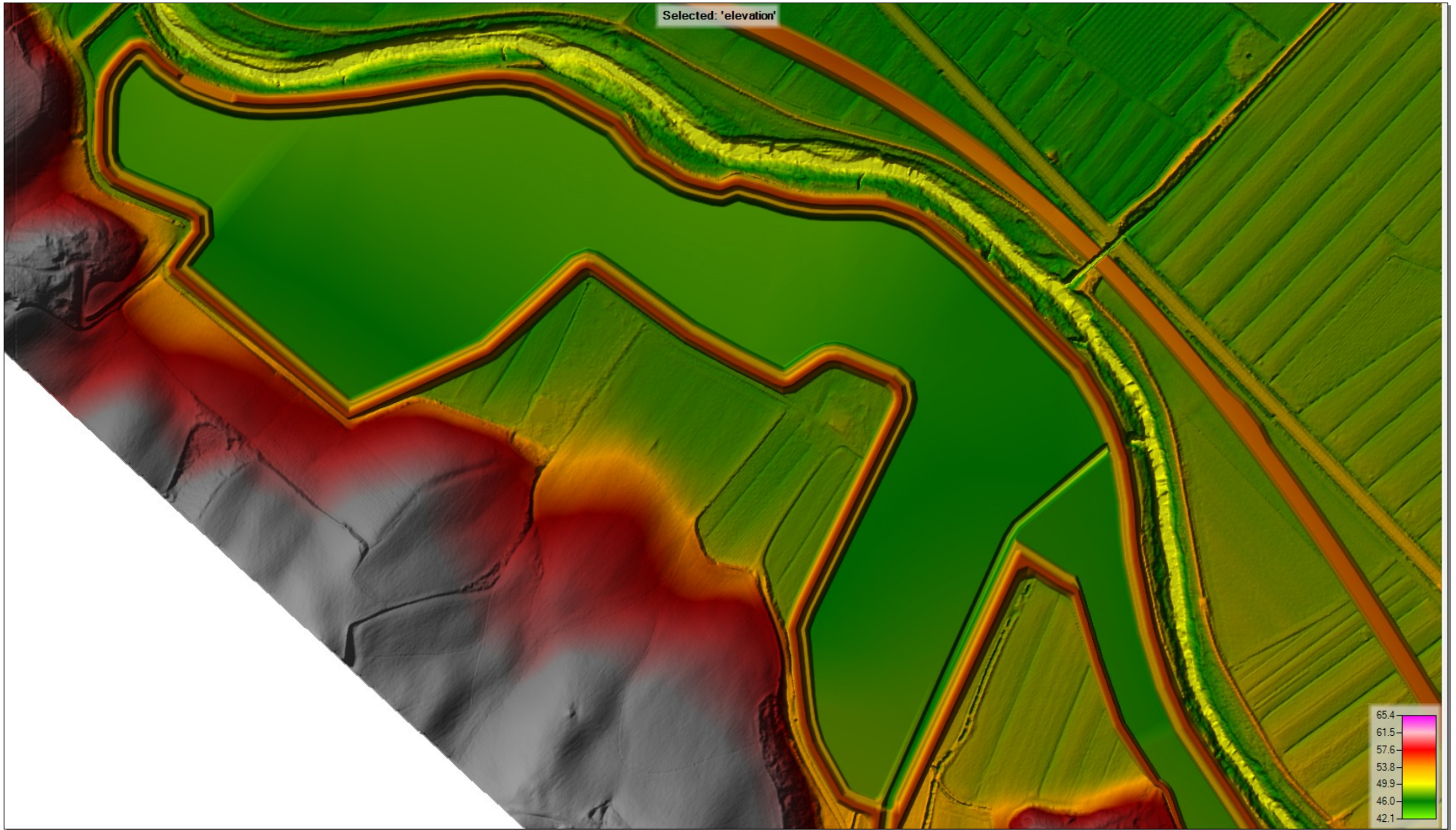
Parte nord della cassa di laminazione – soluzione “SP”
