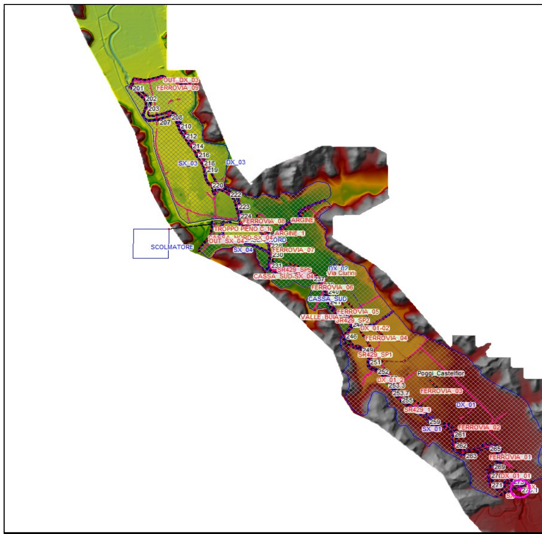
Figura 20 - estensione completa del modello idraulico 2d
