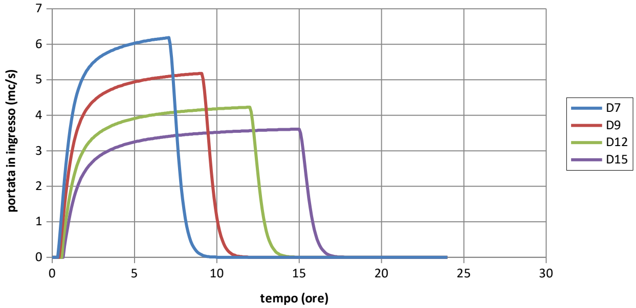
Figura 10 - Idrogrammi del Borro Corniola per Tr30
