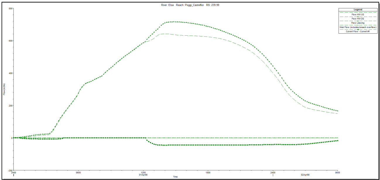
Figura 27 - Funzionamento restituzione Vallebuia per Tr200-12
