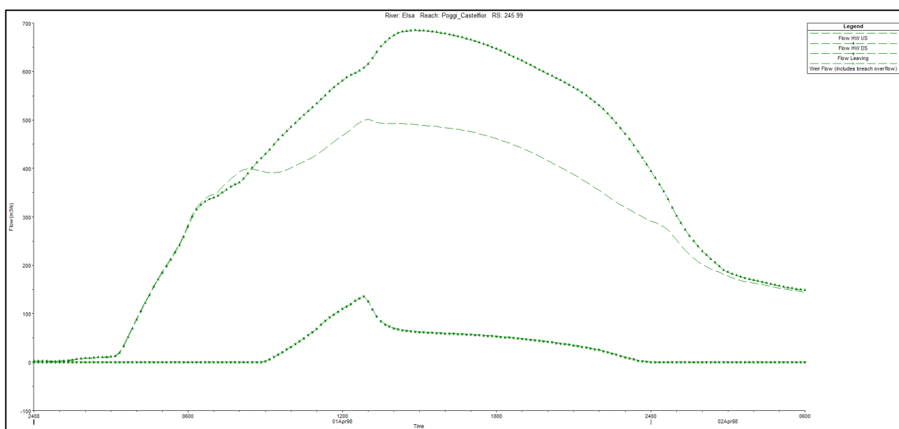
Figura 23 - Funzionamento sfioratore in ingresso per Tr200-12
