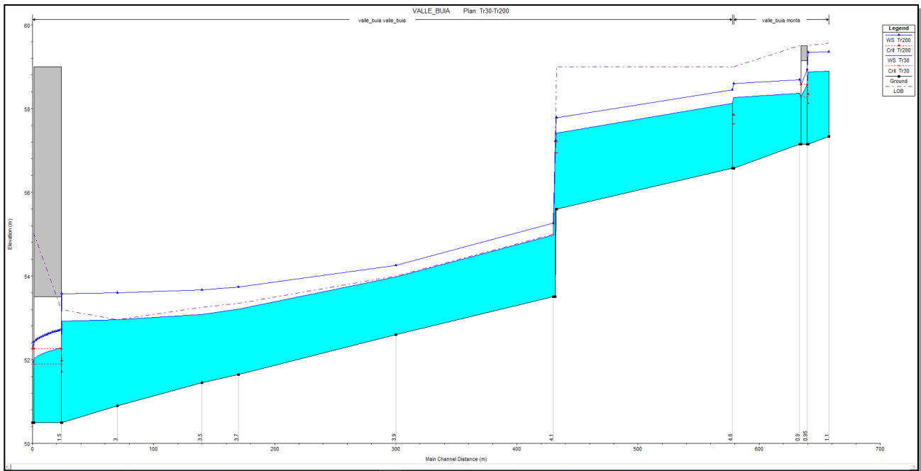
Figura 30 - profilo idraulico Valle Buia per durata critica propria
