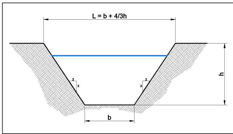
Figura 33 - schema dimensionale del canale di gronda
