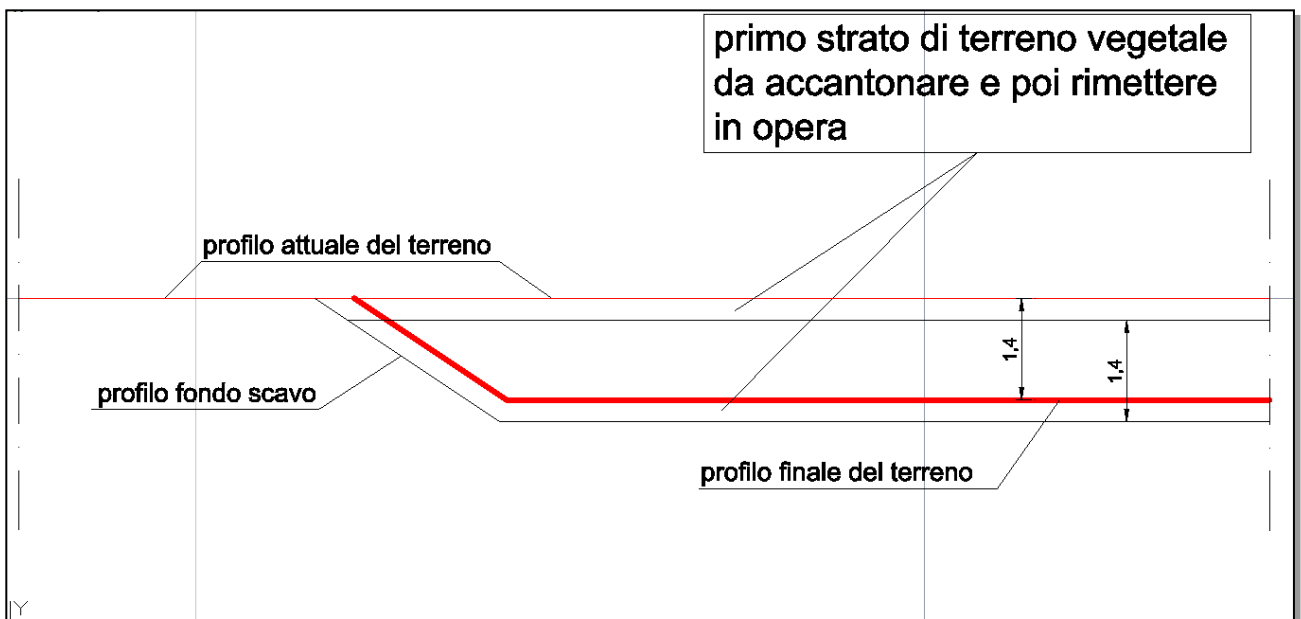
Figura 19 - schema di scavo area di compensazione
