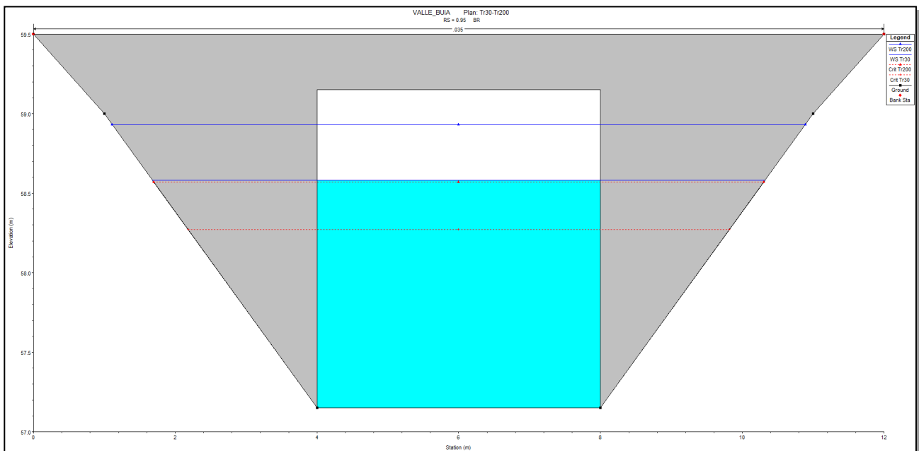
Figura 31 - attraversamento Valle Buia a monte cassa
