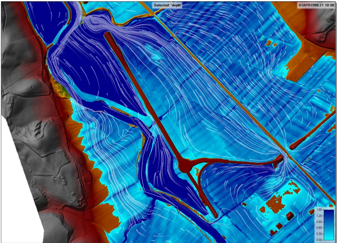
Figura 25 - direzione dei flussi durante la fase critica
