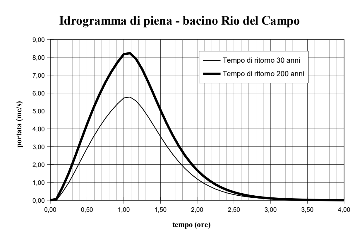
Figura 15 - idrogrammi critici Rio del Campo al Tesoro
