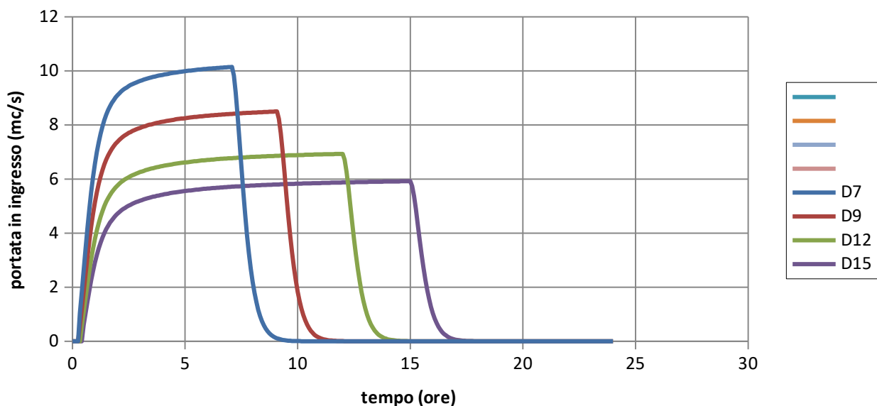
Figura 5 - idrogrammi del Borro Corniola per Tr200
