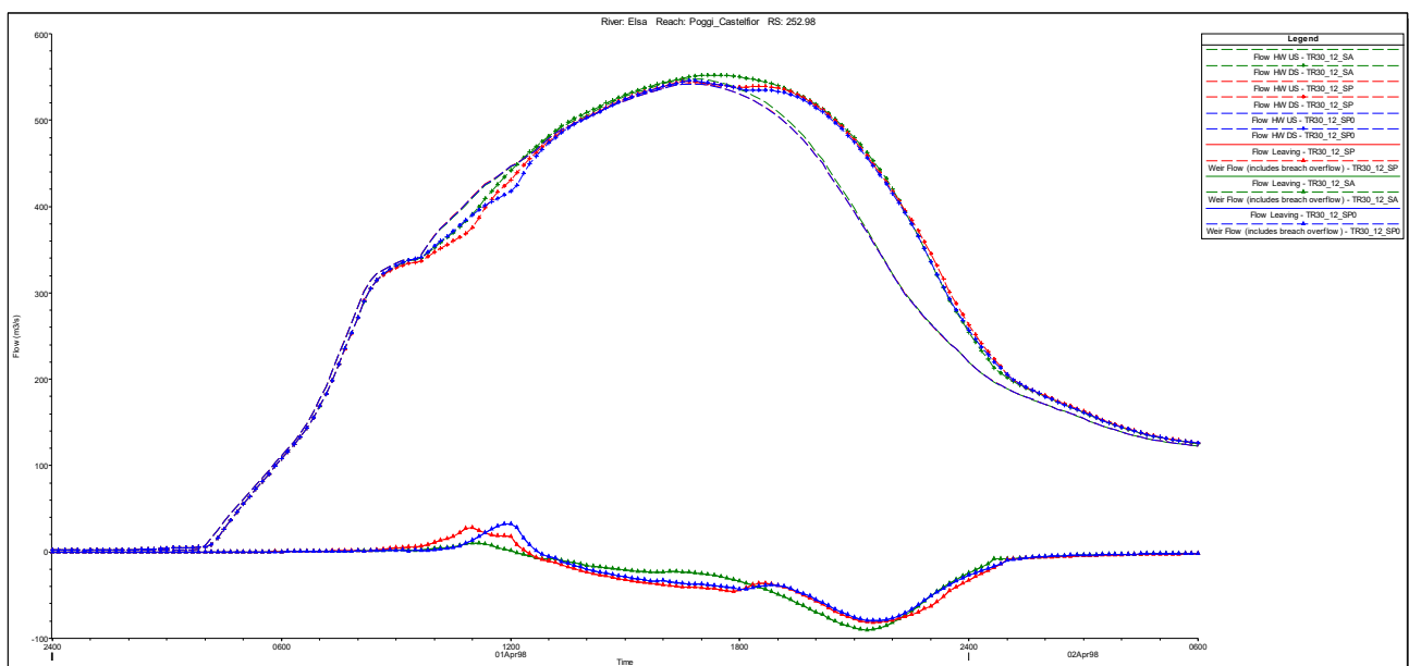
Figura 24 - andamento delle portate in ingresso e uscita dalla sponda opposta allo sfioratore della cassa
