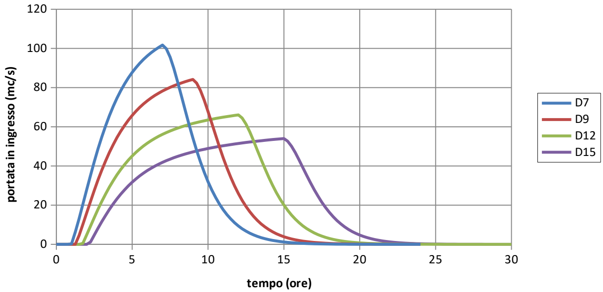
Figura 12 - Idrogrammi del Torrente Pesciola per Tr30
