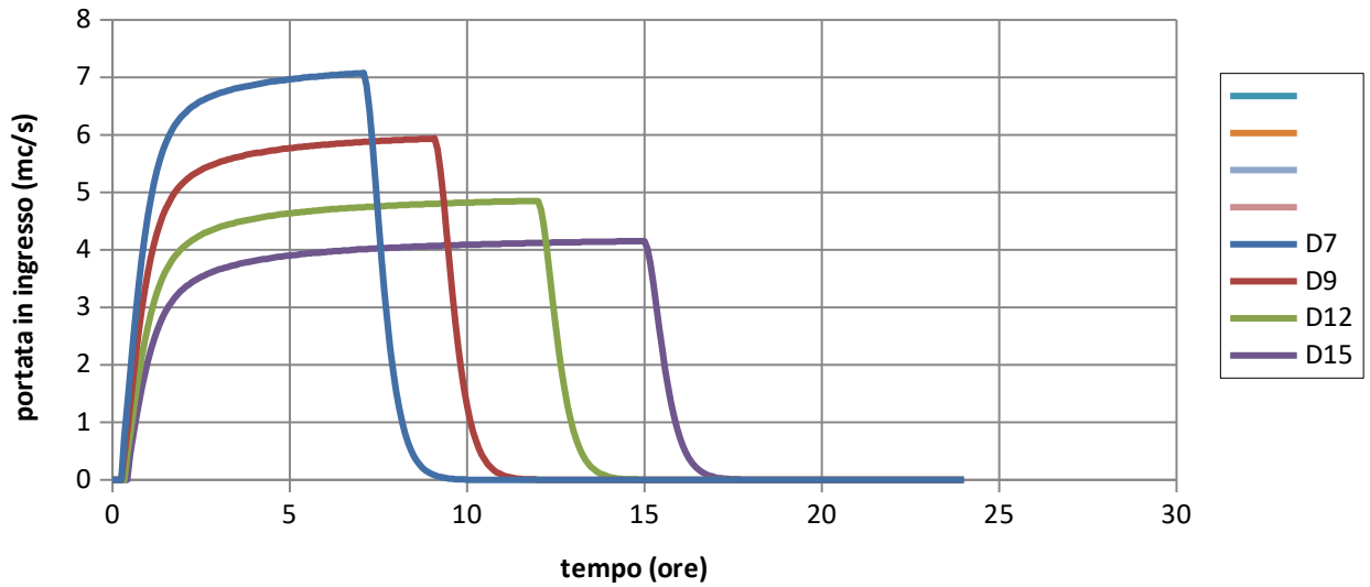
Figura 6 - idrogrammi del Rio Valle Buia e Rio Campo al Tesoro unificati per Tr200
