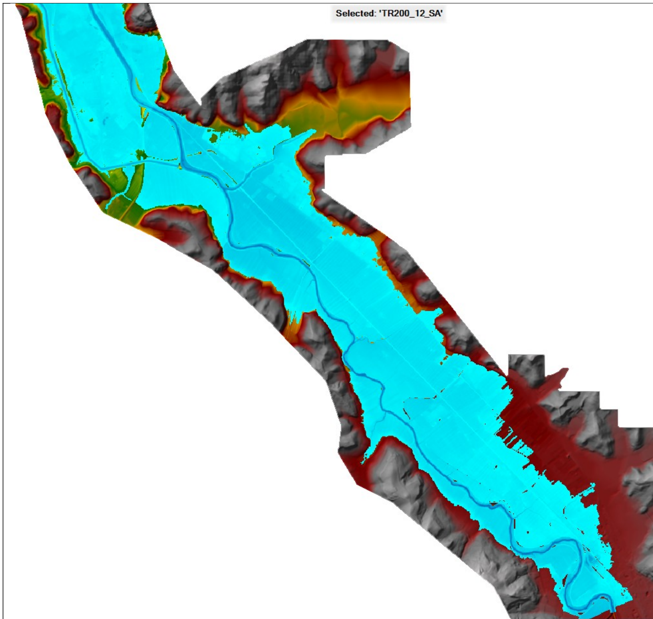
Battenti di inondazione per Tr200 – stato attuale (12 ore)
