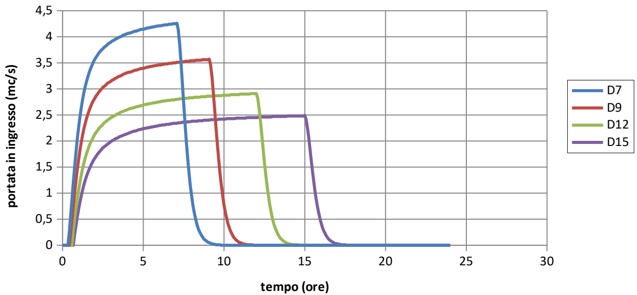
Figura 11 - Idrogrammi del Rio Valle Buia e Rio Campo al Tesoro unificati per Tr30
