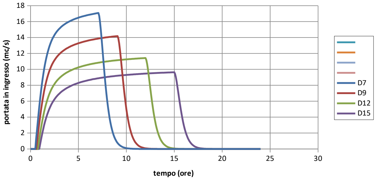
Figura 8 - Idrogrammi del Rio Vallone per Tr200
