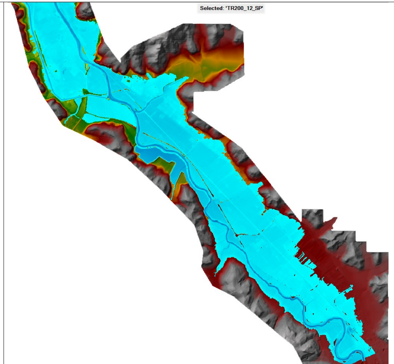
Battenti di inondazione per Tr200 – stato di progetto (12 ore)
