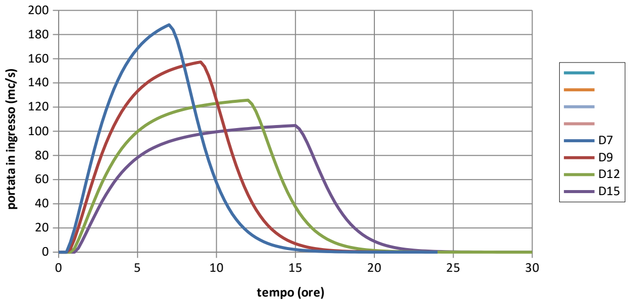
Figura 7 - Idrogrammi del Torrente Pesciola per Tr200
