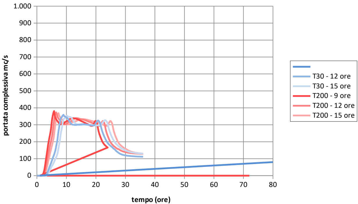
Figura 2 - idrogrammi in ingresso alla sezione di monte - solo parte in alveo
