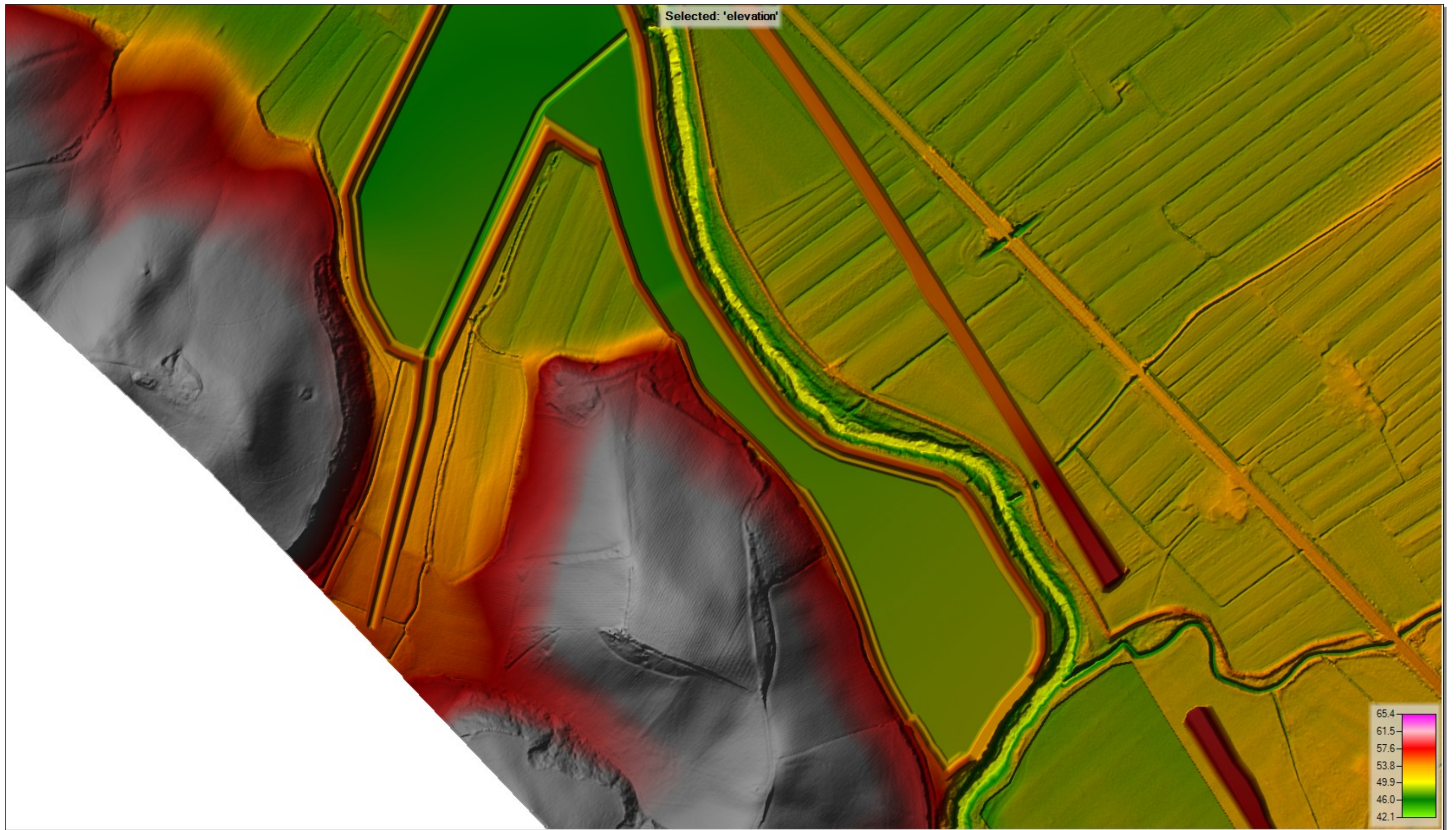
Parte sud della cassa di laminazione – soluzione "SP"
