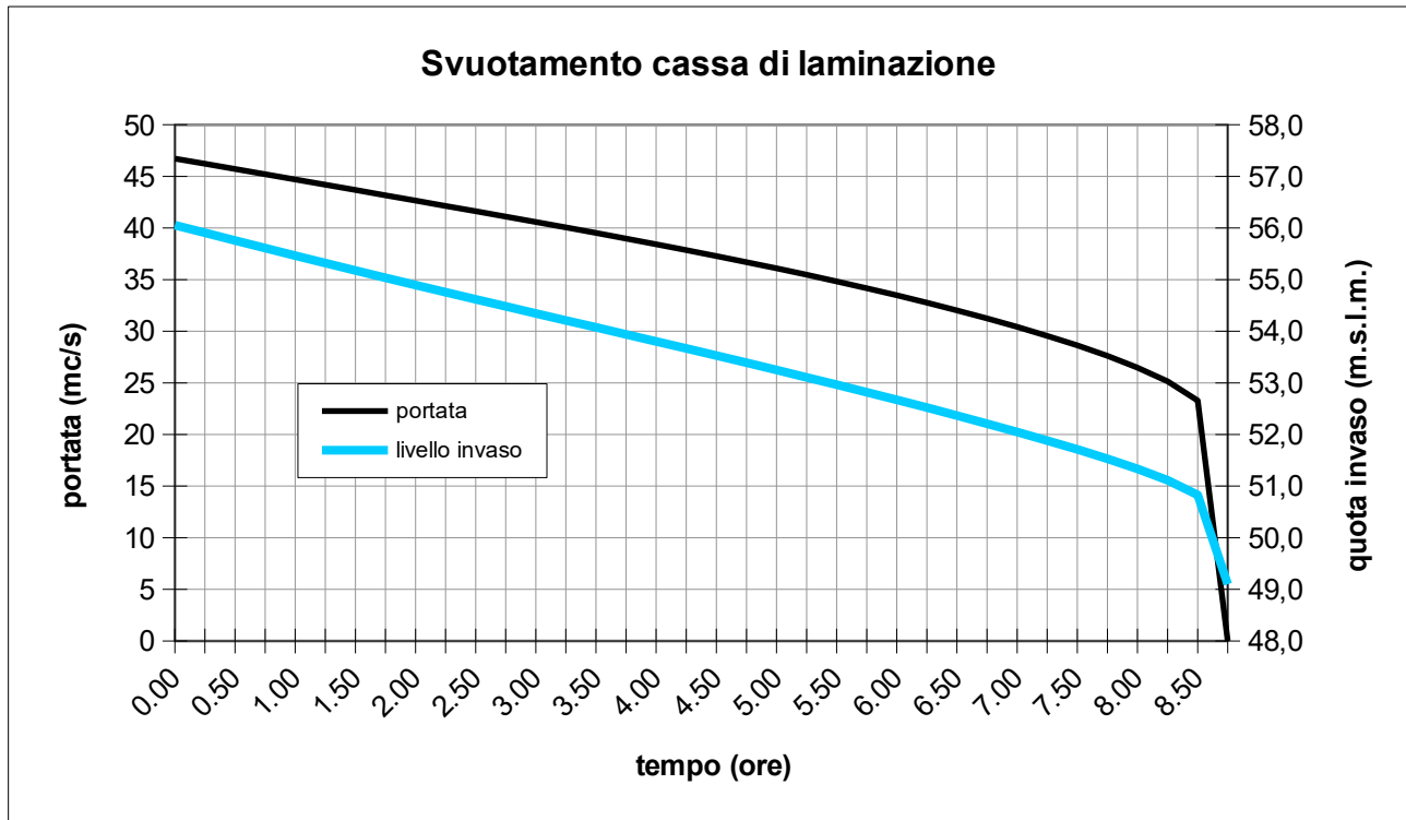
Figura 29 - svuotamento della cassa
