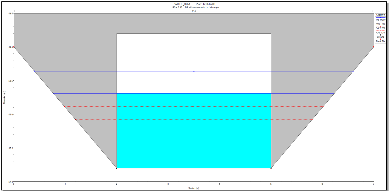
Figura 32 - attraversamento Rio del Campo al Tesoro a monte cassa
