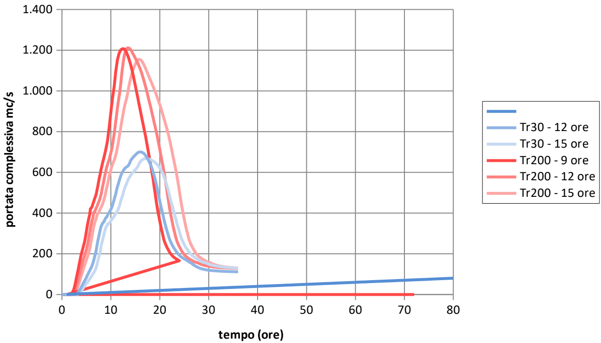
Figura 1 - idrogrammi di ingresso al modello nella sezione di monte
