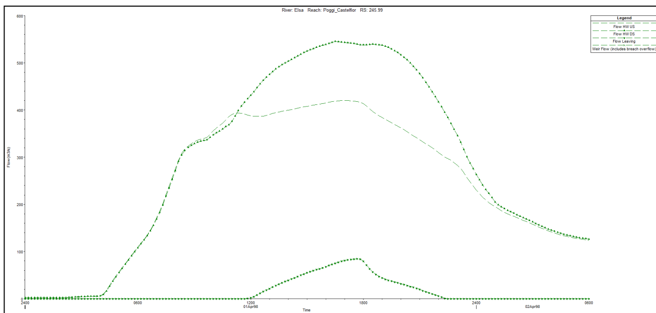
Figura 22 - Funzionamento sfioratore in ingresso per Tr30-12
