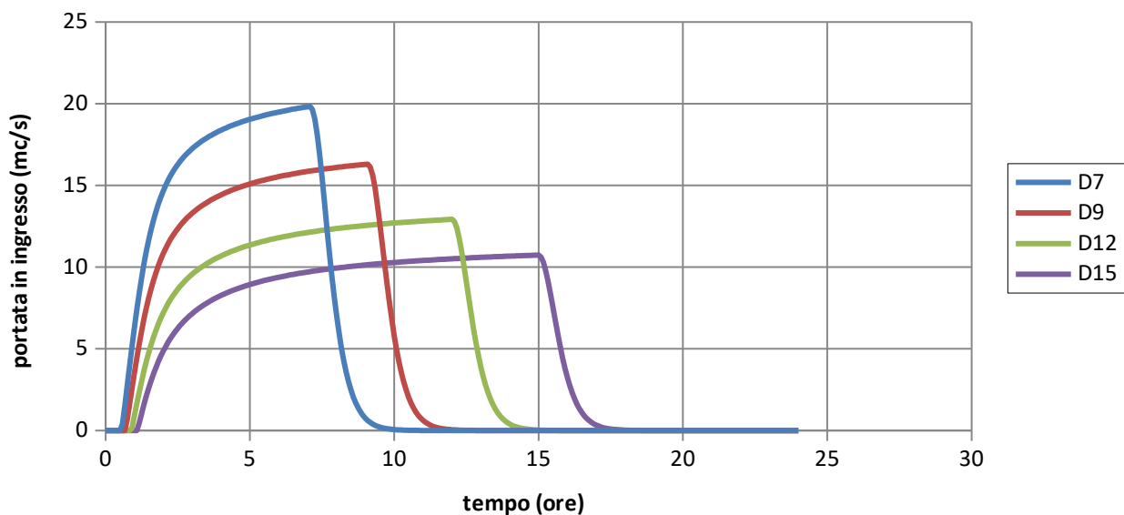
Figura 4 - idrogrammi del Borro Renaccio per Tr200
