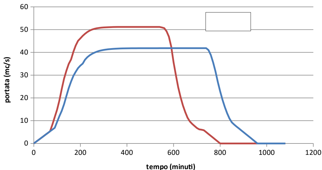
Figura 17 - idrogrammi provenienti da Rio Pietroso e Rio Arnese
