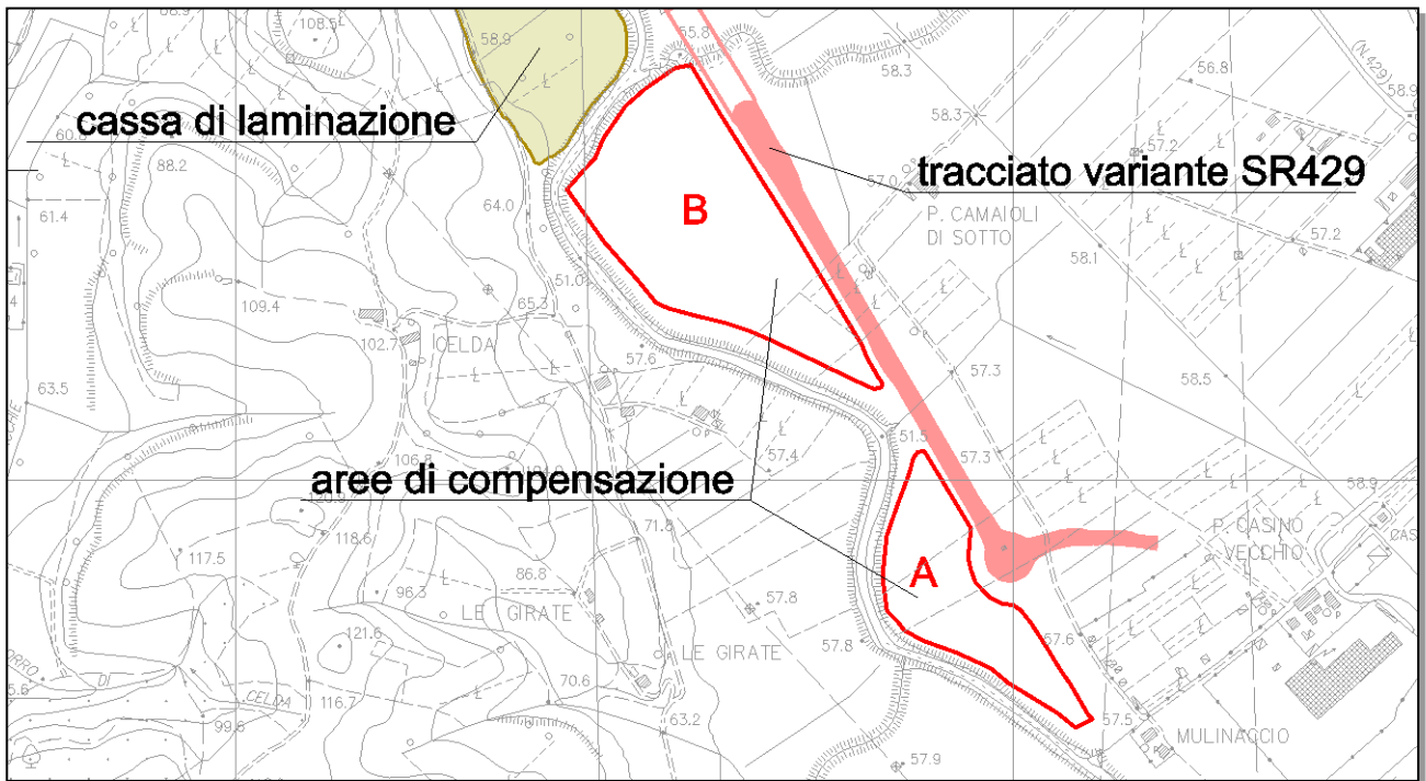
Figura 18 - ubicazione aree di compensazione
