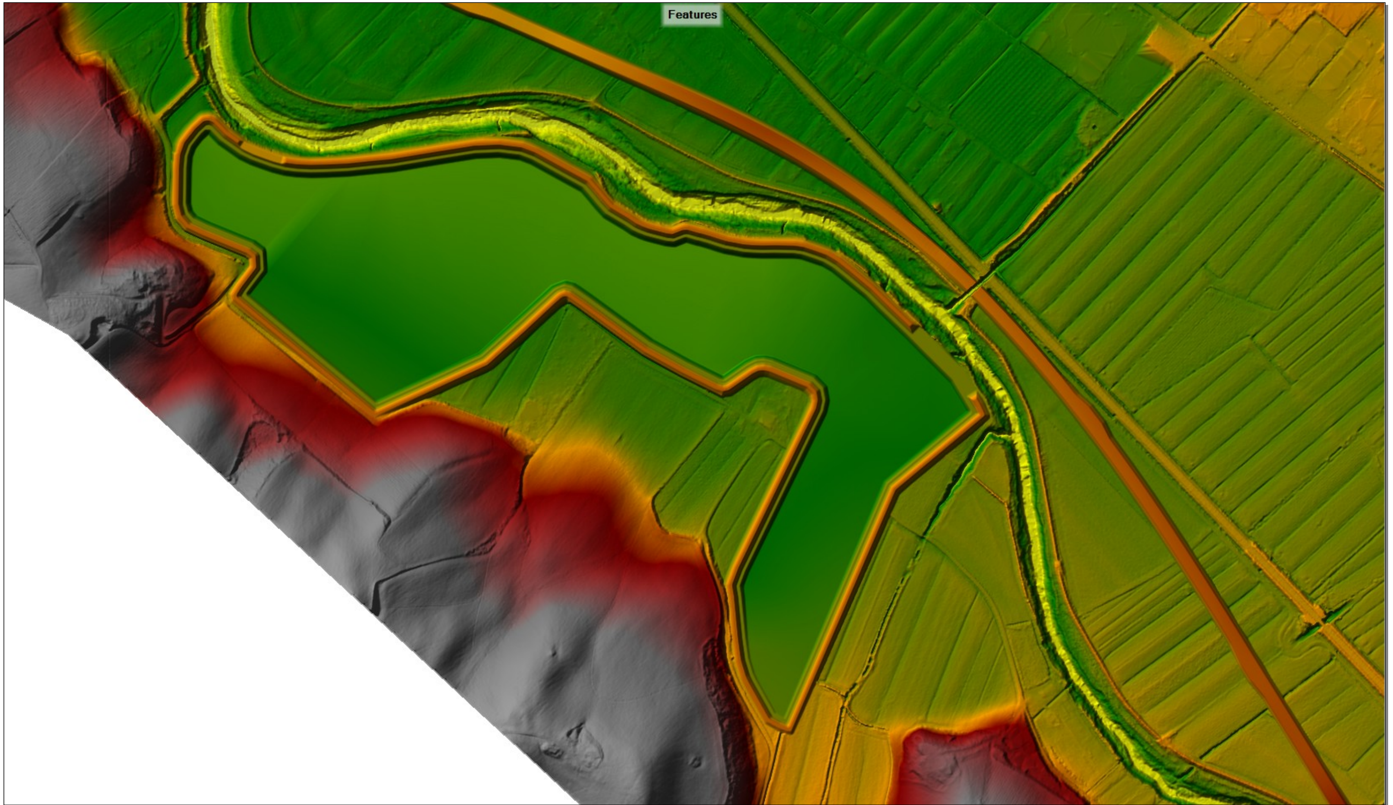
Cassa di laminazione – soluzione "SPG"
