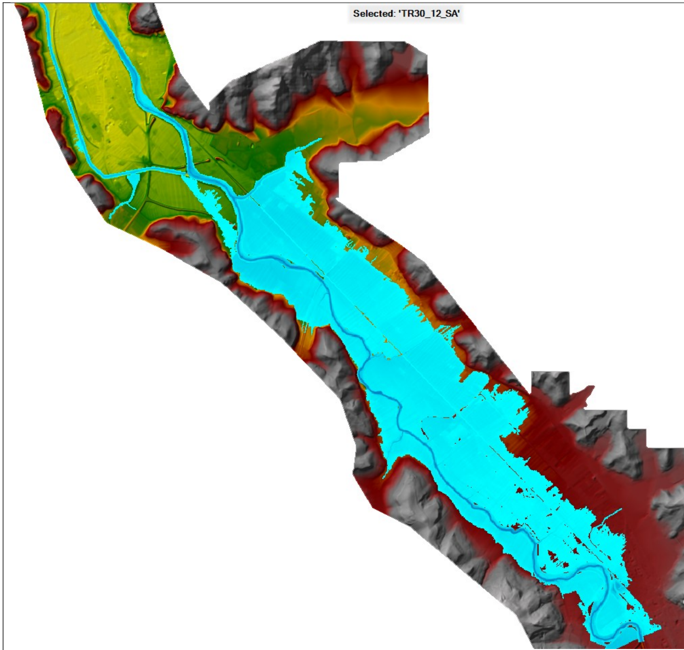
Battenti di inondazione per Tr30 – stato attuale (12 ore)
